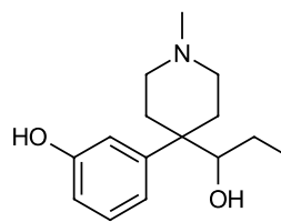
pelkistystuote
